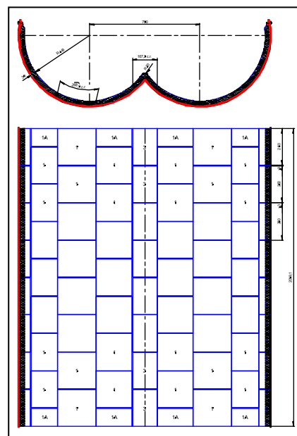
Vyložení míchačky „Forberg“
