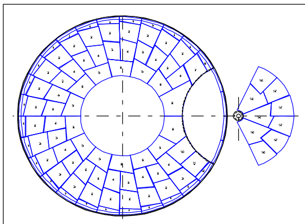
Výkres přesného vyložení míchačky betonových směsí „RTM“
