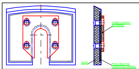
Lopátka s podkladovým plechem
