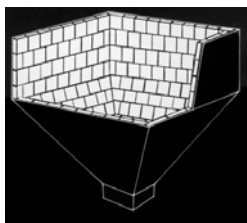
Schéma vyložení násypky
