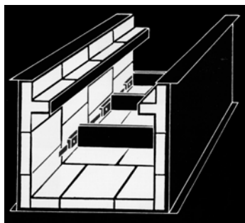
Řetězový dopravník vyložený taveným čedičem nebo eucorem
