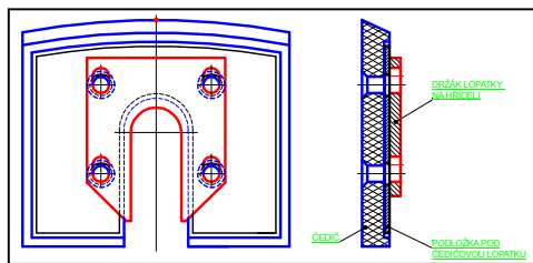
Lopatka s podkladovým plechem
