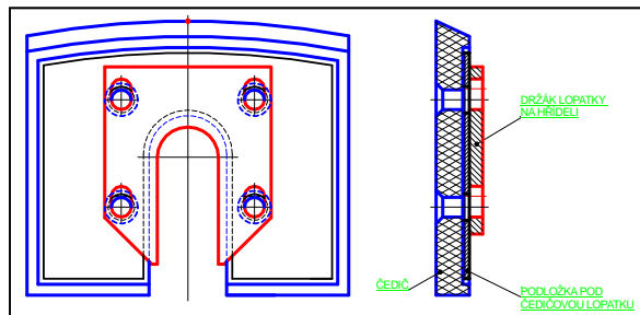
Lopatka s podkladovým plechem
