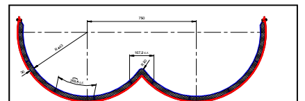
Eucorové vyložení míchačky - výpust'
