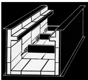
Řetězový dopravník vyložení taveným čedičem nebo eucorem
